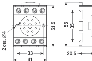
Клеммная колодка
